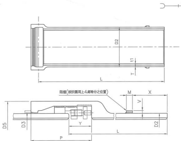
■ 接合部詳細
